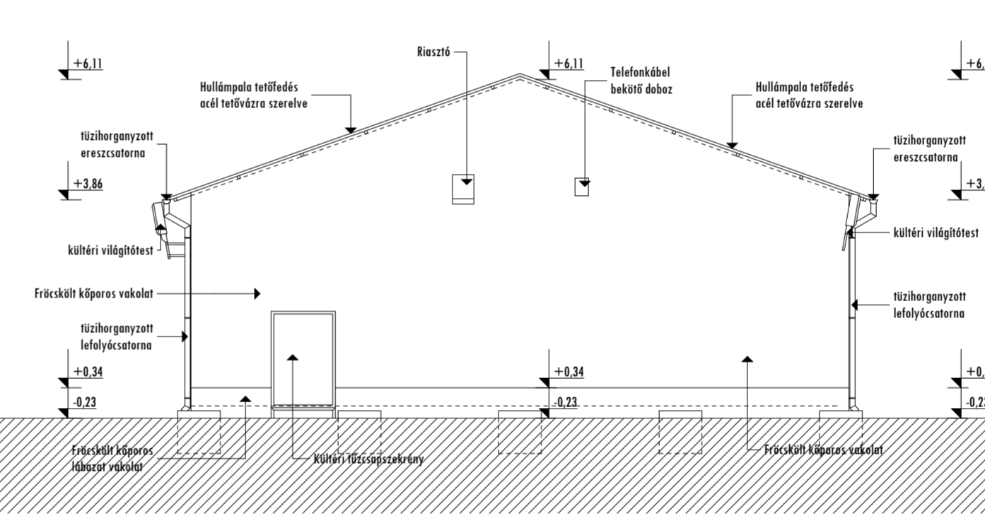
DÉLI HOMLOKZAT M 1:100
