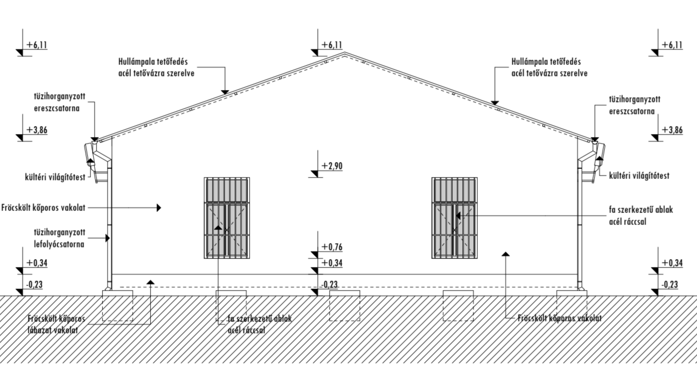
ÉSZAKI HOMLOKZAT M 1:100
