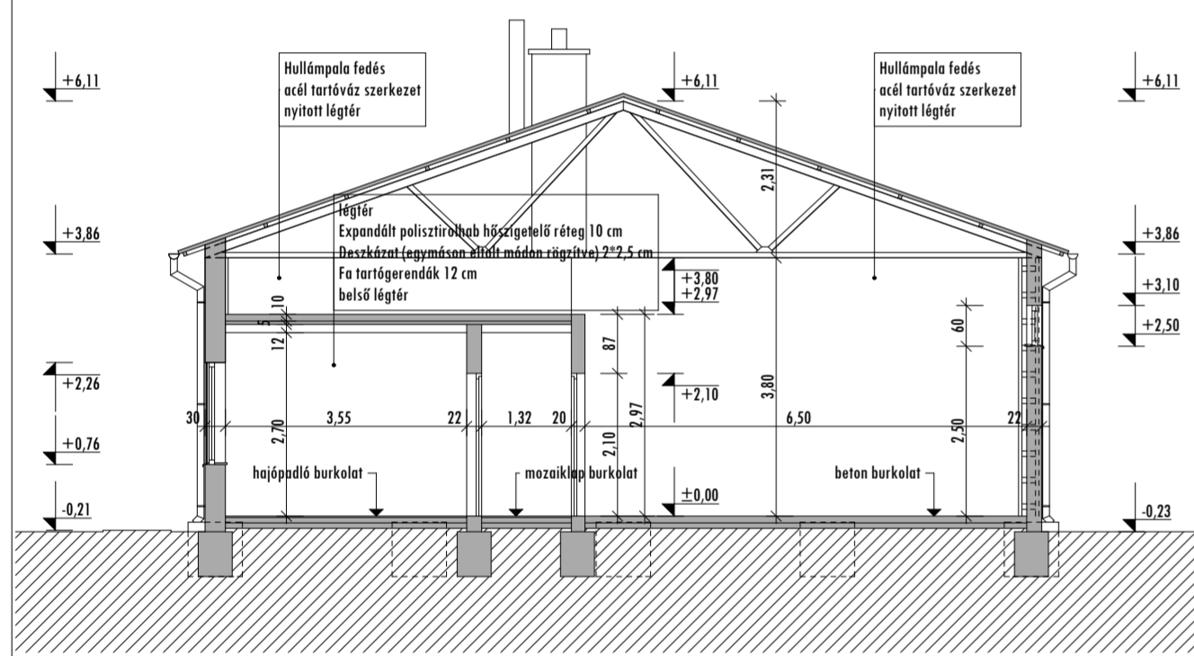
A-A METSZET M 1:100
